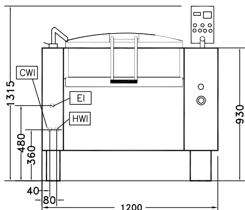
Zepředu
